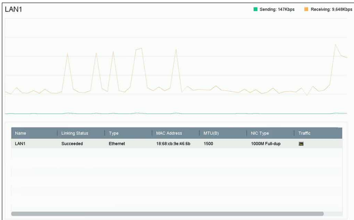
図 15-2 ネットワークトラフィック
