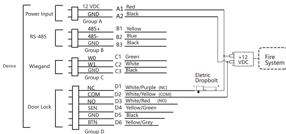
図 4-3 配線デバイス
