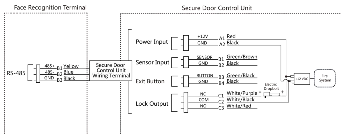
図4-4 ワイヤ固定ドア制御ユニット
