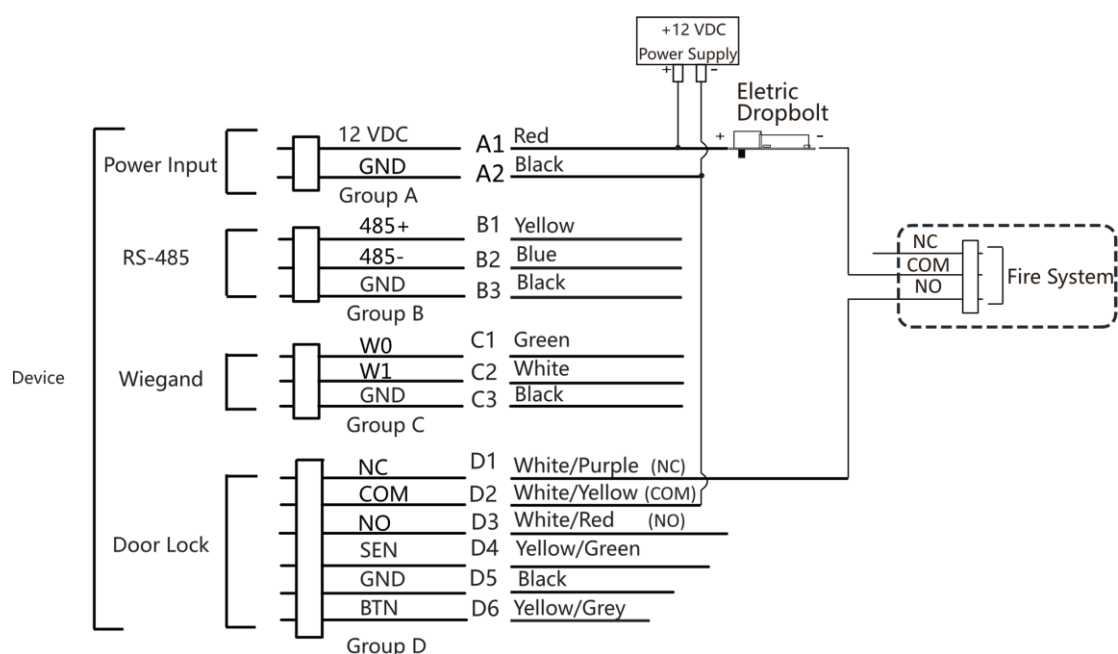
図 4-5 配線装置
