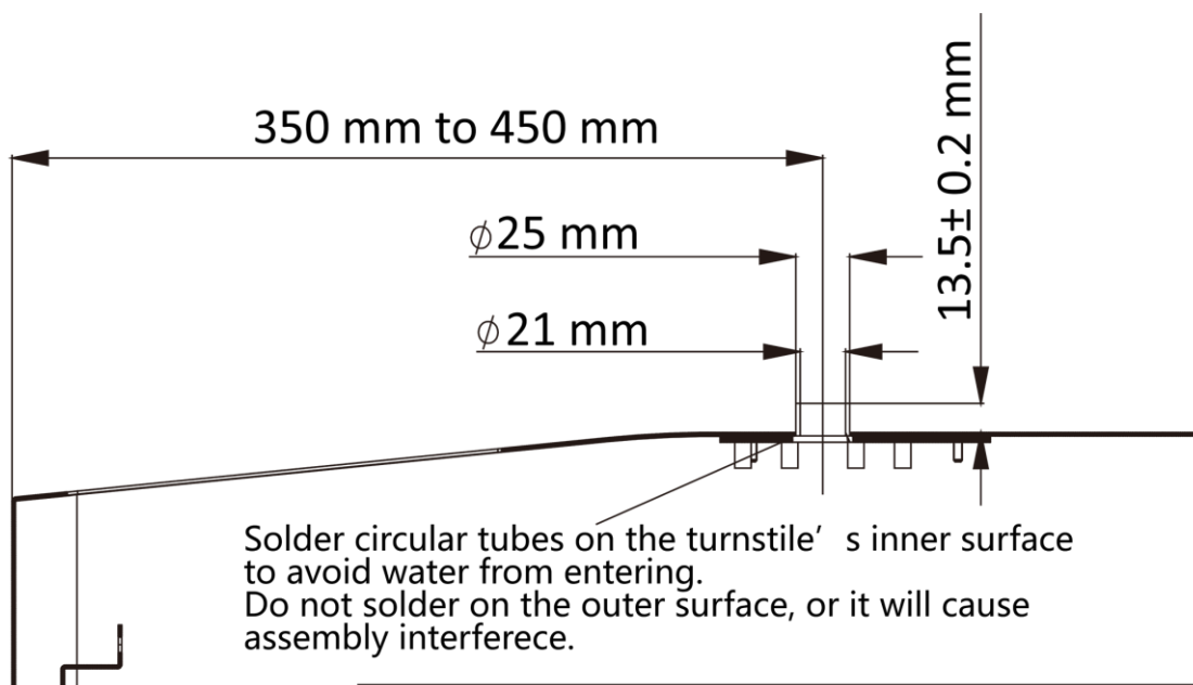
図3-17 チューブのはんだ付け
