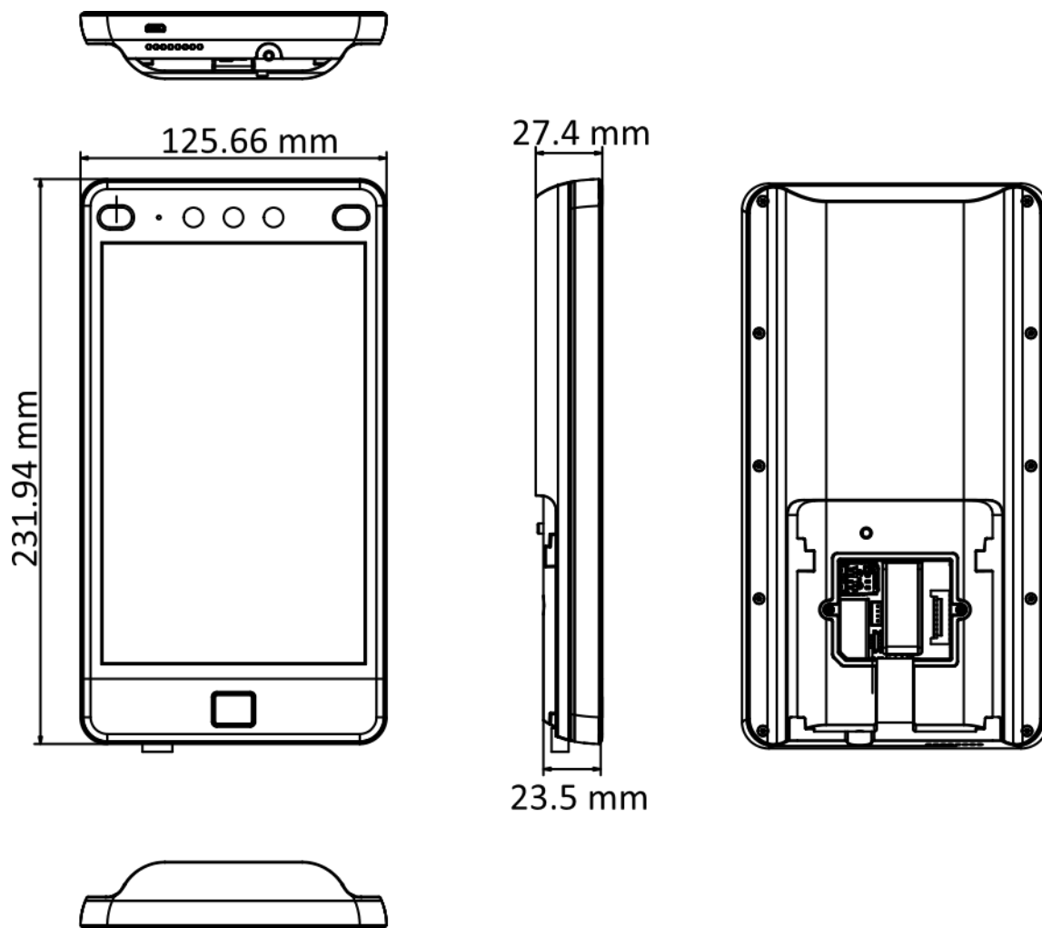
図 D-1 寸法
