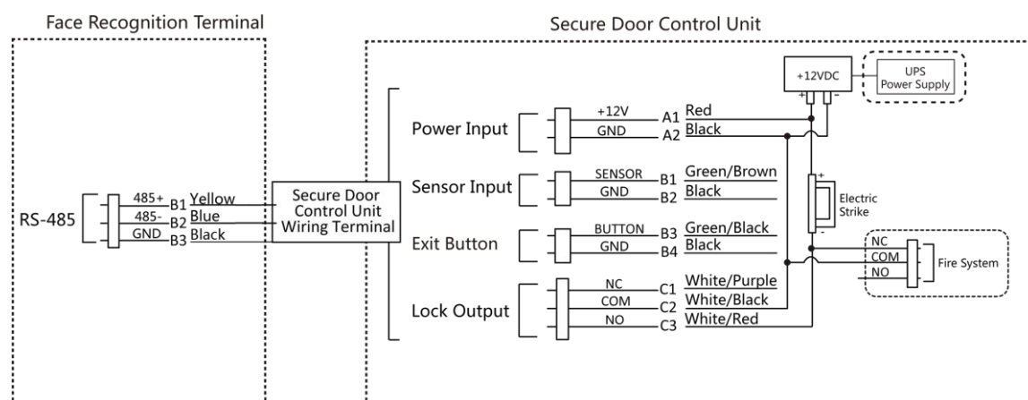
図4-8 配線図
