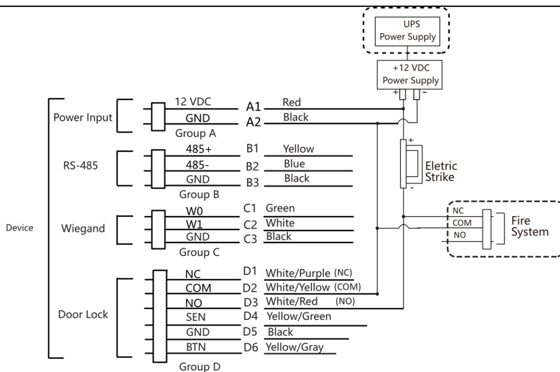
図4-7 装置配線図
