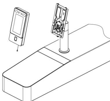
図3-15 装置の固定
