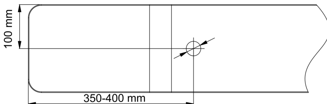
図3-10 回転式改札機の穴あけ
