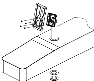
図 3-14 取付テンプレートの固定
