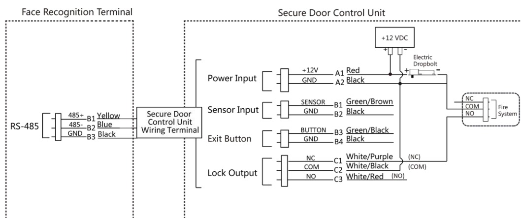
図4-6 配線 セキュアドア制御ユニット
